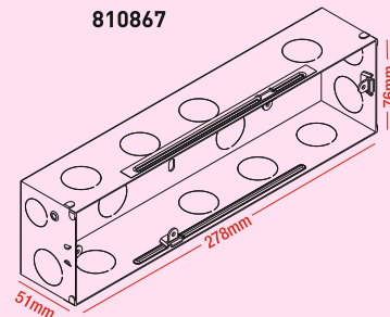
9 module 810867
