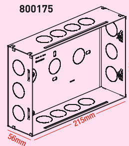
12 module 800175
