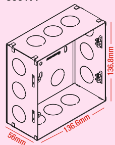
8 module (Vertical) 800177
