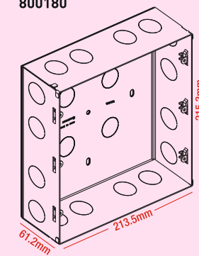
18 module 800180
