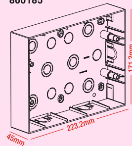
12 module 800185
