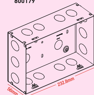
16 module 800179
