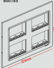
12 module 800165
