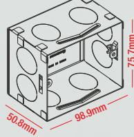
3 module 800173
