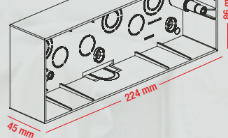
6 module 800186
