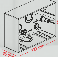
3 module 800183
