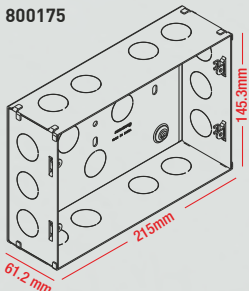
12 module 800175
