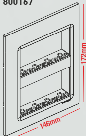
8 module (Vertical) 800167
