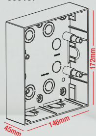
8 module (Vertical) 800187
