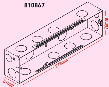
9 module 810867
