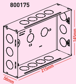
12 module 800175
