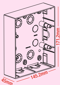
8 module (Vertical) 800187
